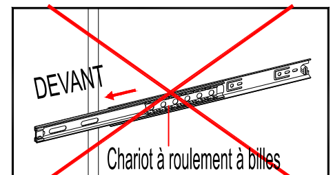
Installation du tiroir de rangement
