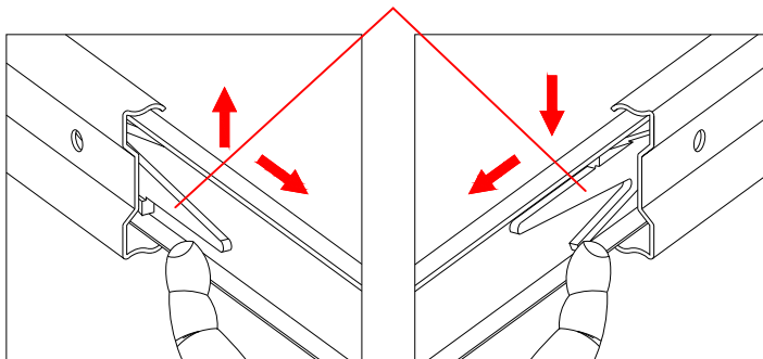
Para remover cajón
